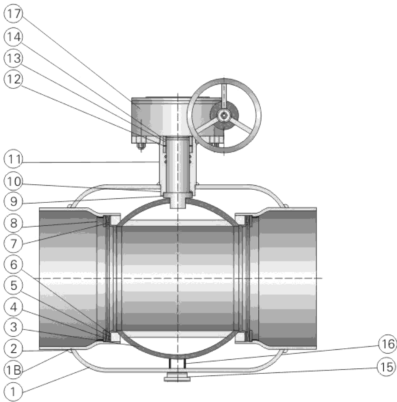
断面図
